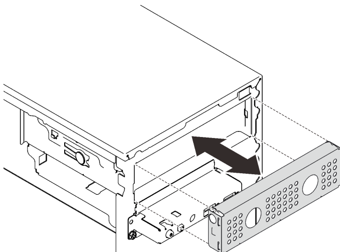
图 55. 安装硬盘插槽保护罩
