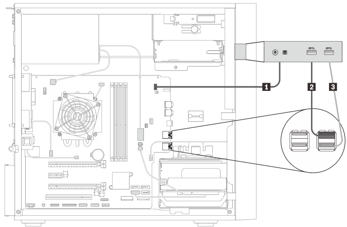
图 24. 前面板的线缆布放
