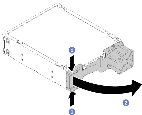
图 52. 打开适配器组合件的滑锁
