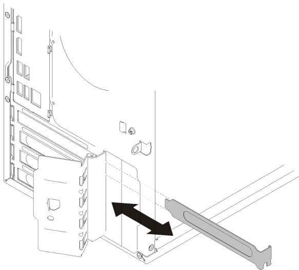
图 99. 卸下 PCIe 适配器支架
