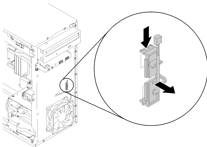
图 114. 卸下热传感器
