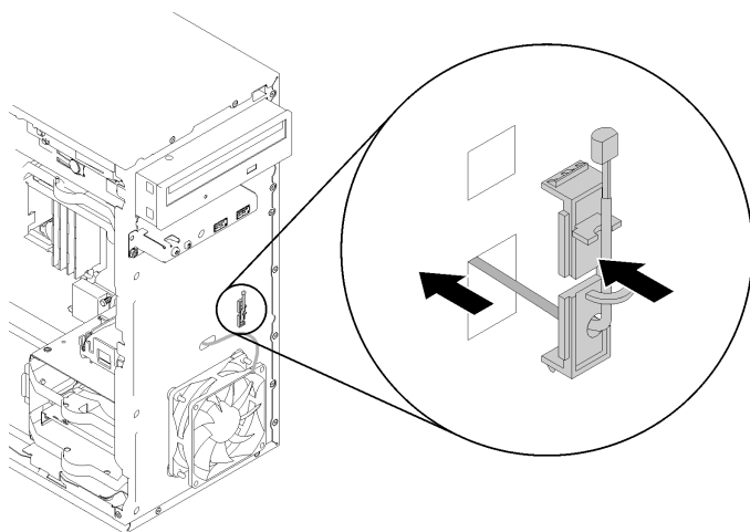
图 115. 安装热传感器
