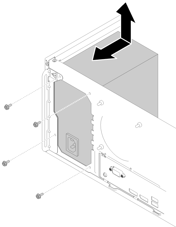
图 103. 安装电源模块单元
