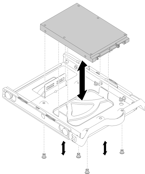
图 37. 从固定器卸下 2.5 英寸硬盘
