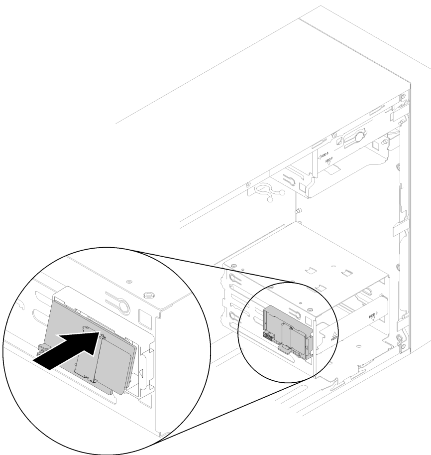
图 69. 安装双 SD 卡适配器
