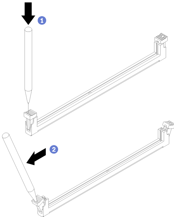
图 31. 打开 DIMM 固定夹
