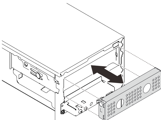
图 45. 安装硬盘插槽保护罩
