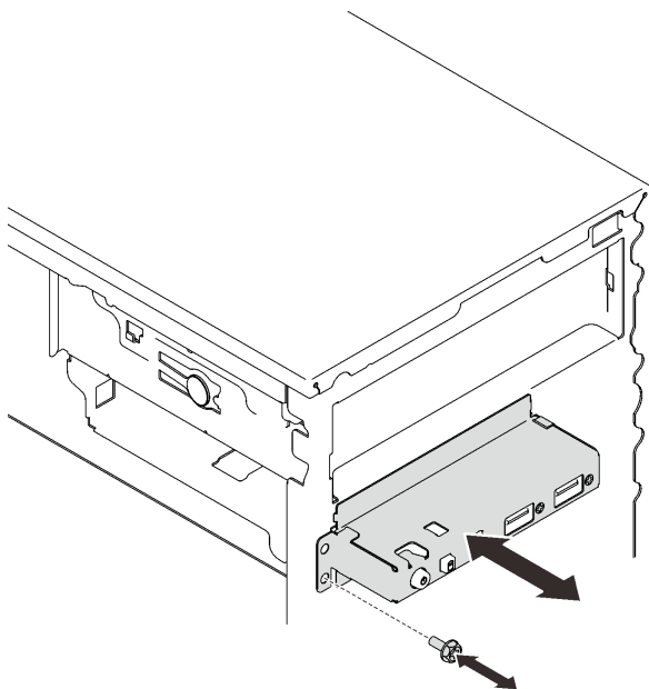
图 86. 安装前面板
