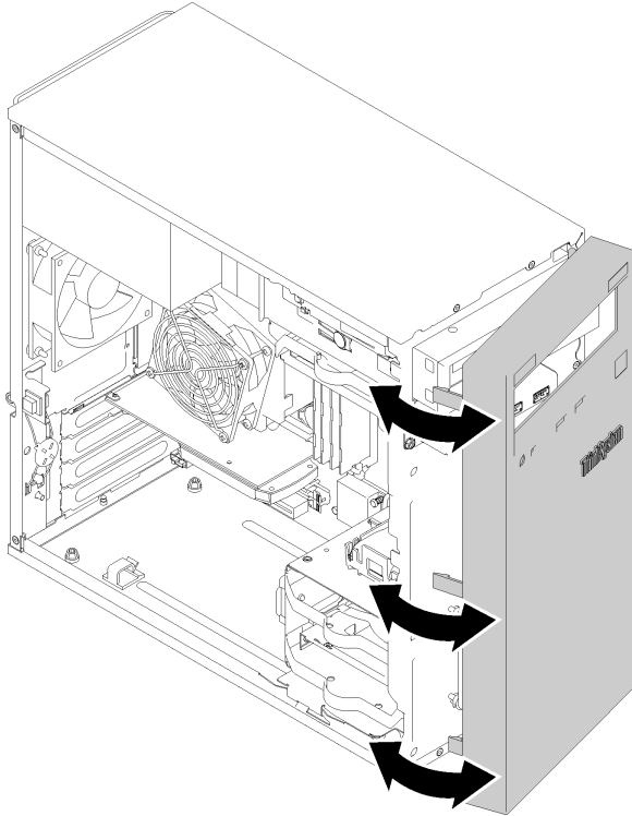
图 83. 安装前挡板
