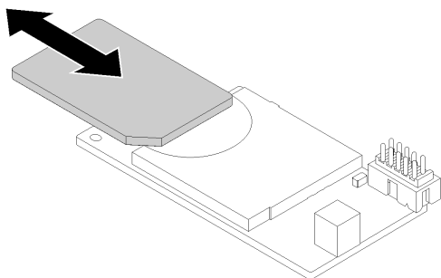
图 68. 将 SD 卡装入双 SD 卡适配器
