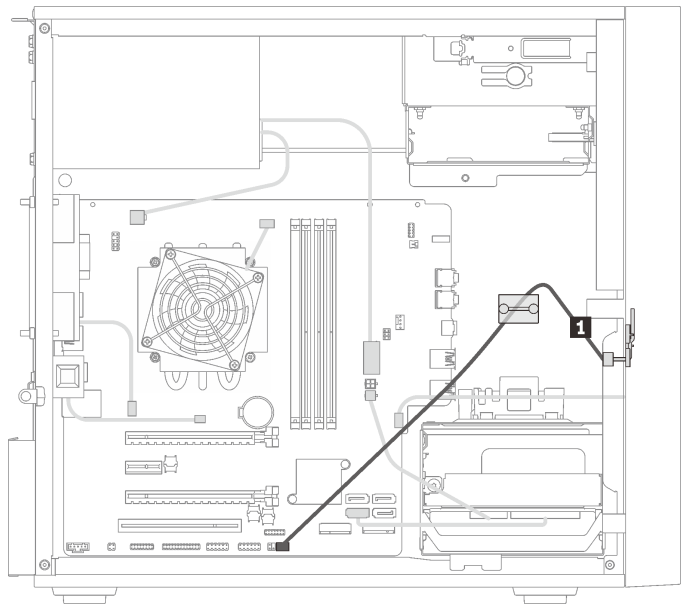
图 25. 热传感器的线缆布放
