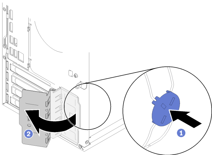
图 98. 打开 PCIe 适配器固定器
