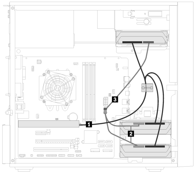
图 20. 三个带有 RAID 适配器的硬盘的线缆布放
