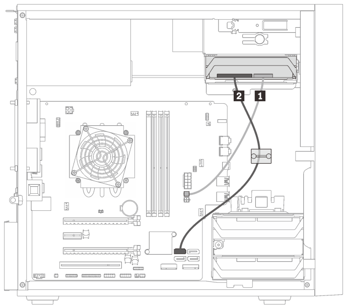
图 13. 硬盘插槽 3 的线缆布放
