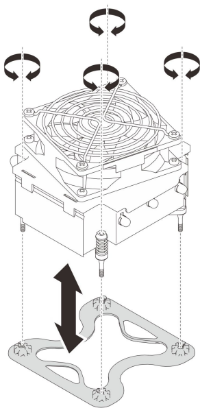
图 89. 卸下框架
