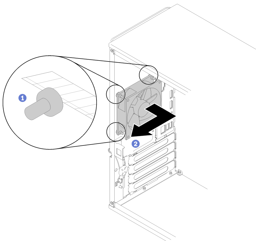
图 74. 卸下背面风扇
