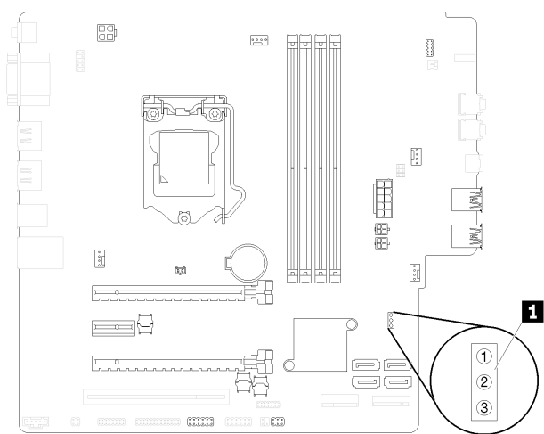
图 7. 主板跳线
