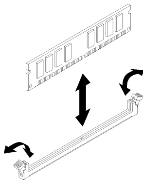
图 30. 卸下 DIMM
