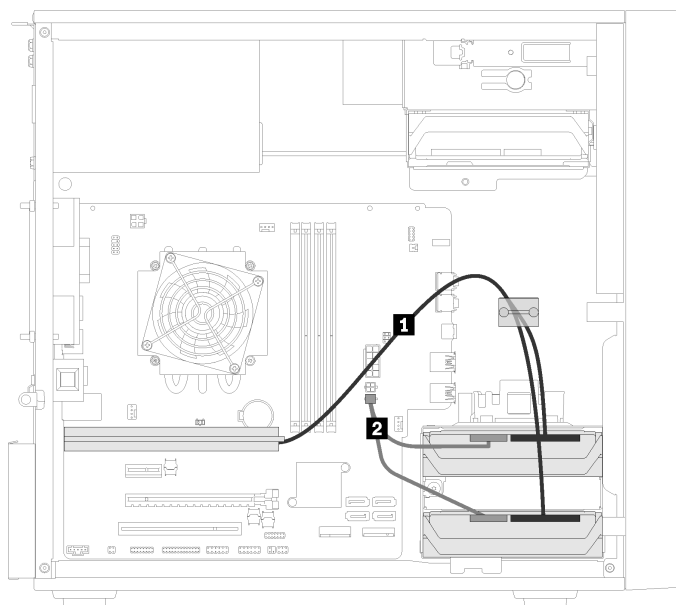
图 19. 两个带有 RAID 适配器的硬盘的线缆布放
