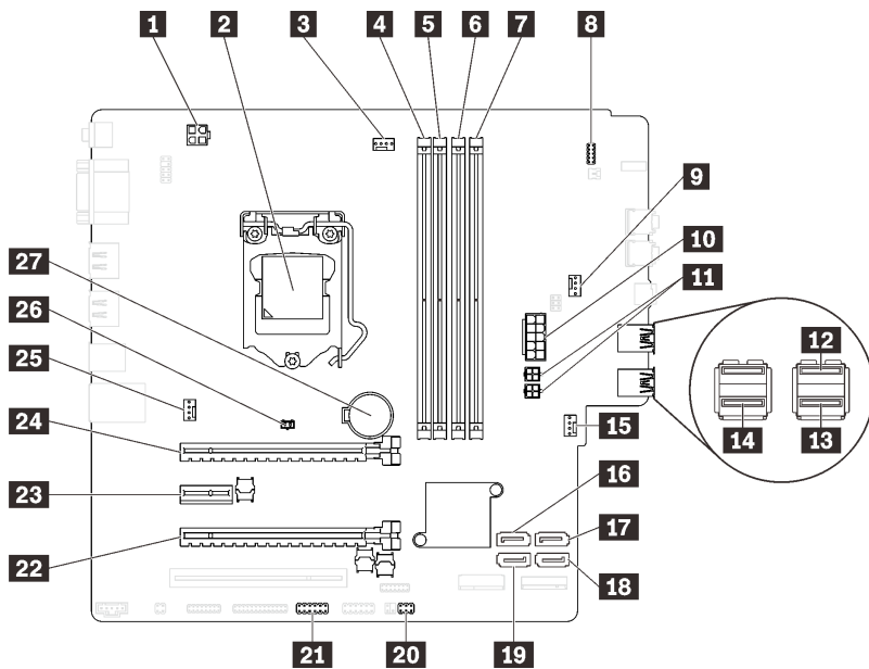
图 6. 主板组件
