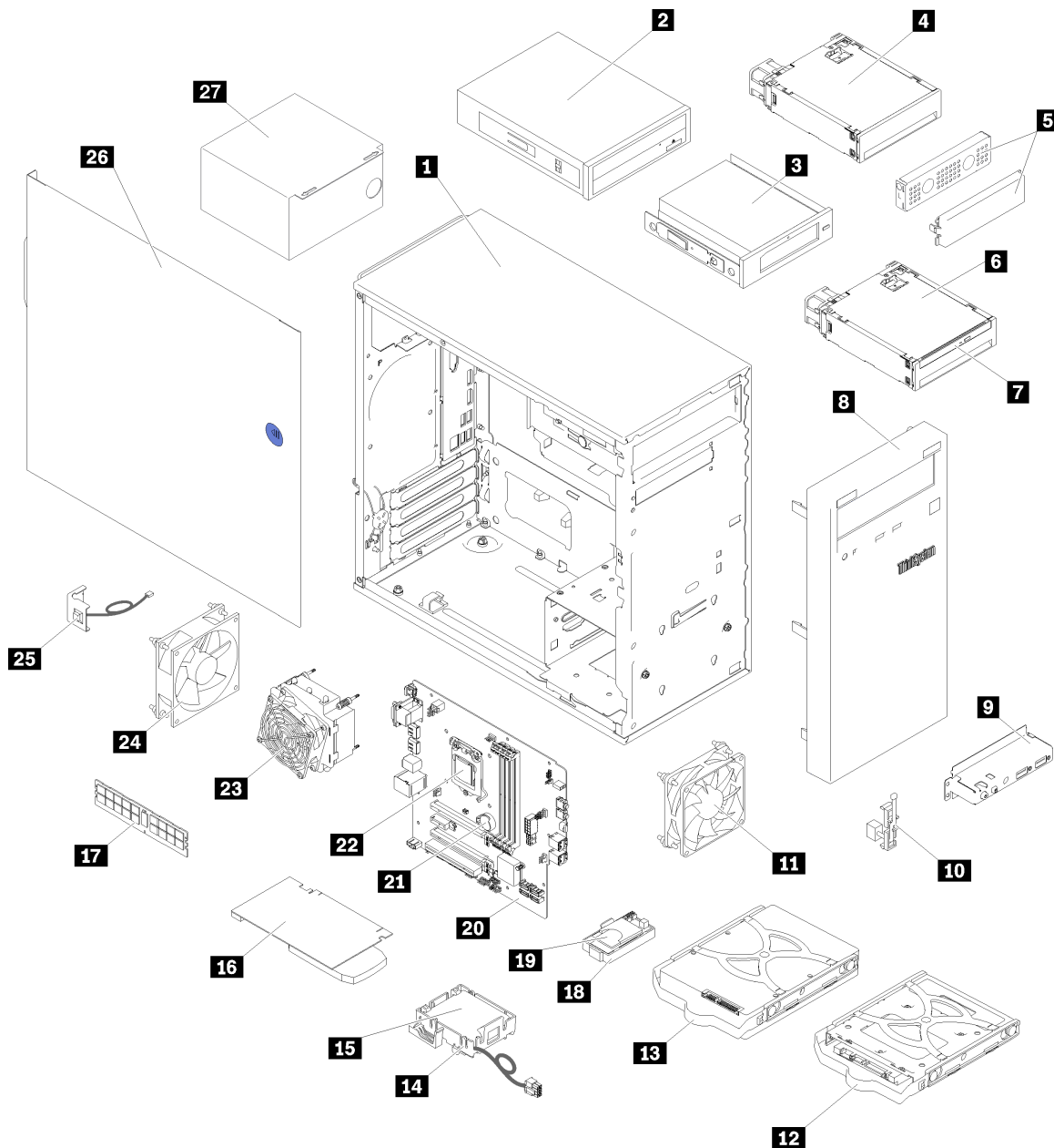
图 26. 服务器组件
