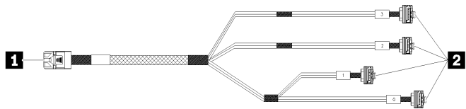
图 17. Mini SAS HD 转 4 SATA 7 针线缆
