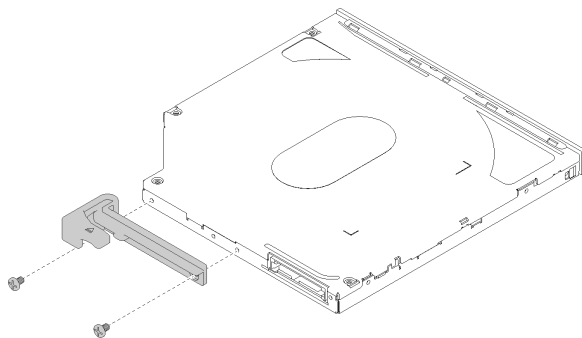
图 57. 将固定器安装到薄型光驱
