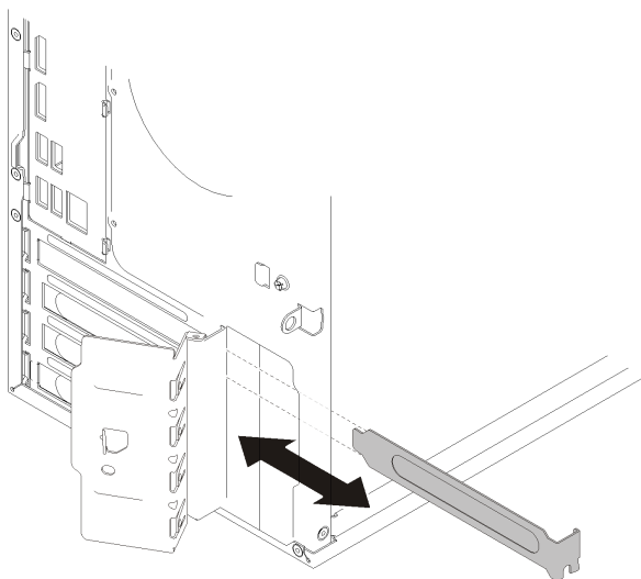
图 97. 安装 PCIe 适配器支架
