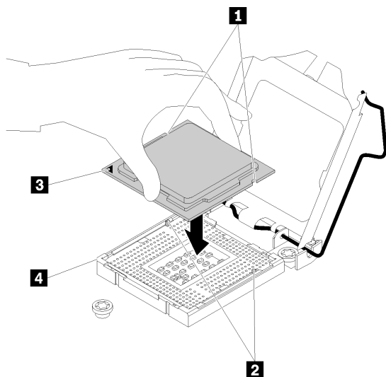
图 107. 安装处理器
