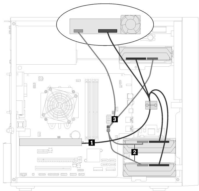
图 21. 四个带有 RAID 适配器的硬盘的线缆布放
