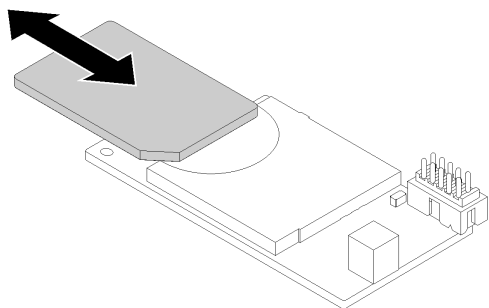
图 65. 从双 SD 卡适配器中卸下 SD 卡
