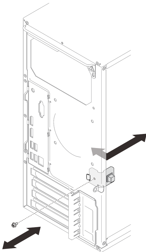
图 94. 安装机箱入侵感应开关
