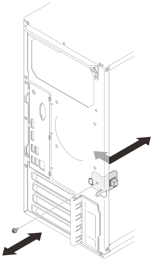
图 93. 卸下机箱入侵感应开关
